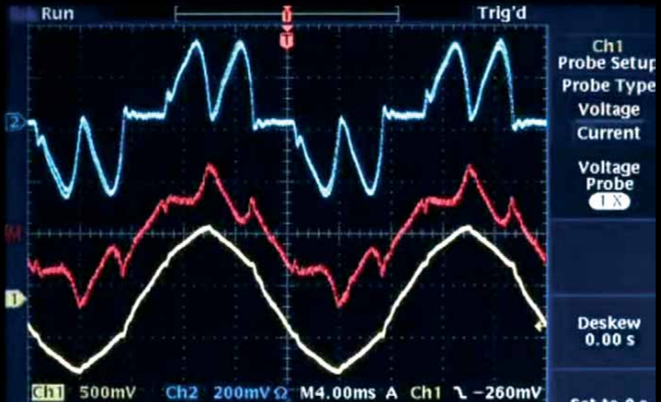
Filtry aktywne monitorują i analizują odkształcenie. Prąd korekcyjny filtra jest generowany w przeciwfazie aby wyeliminować żądane odkształcenie.
